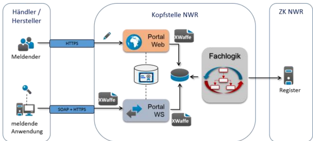
Abbildung 1 Architektur der NWR-Kopfstelle für Händler und Hersteller
